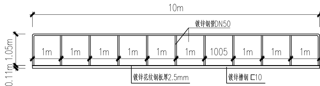
钢板桥栏杆图
