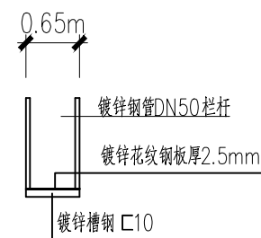
钢板桥侧面图
