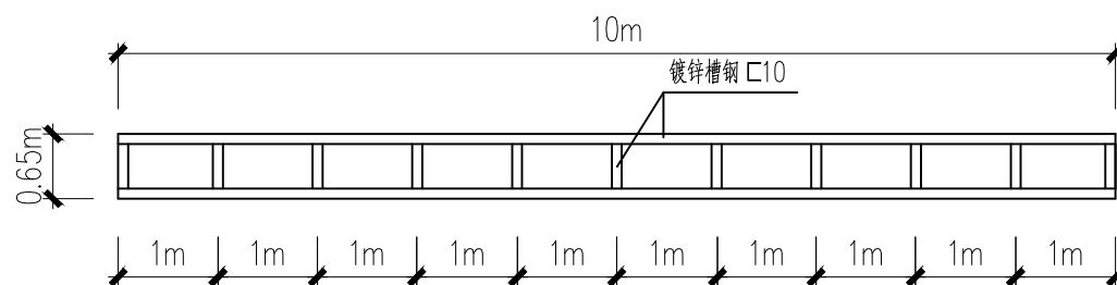
钢板桥面结构图
